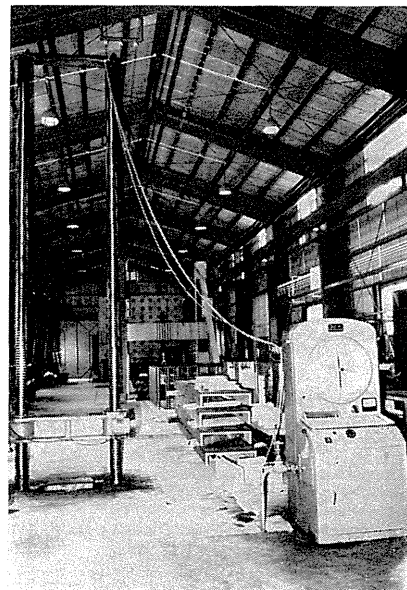
写真-2.3 100 ton 長柱圧縮試験機
