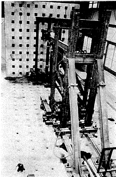
写真-2.2 構造物試験台（耐荷能力 200 ton）
