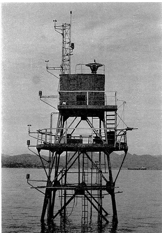
写真-2・21 観 測 塔
