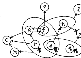
与併存到達図
