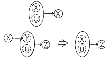
図 1. 射影則と擬似推移則
