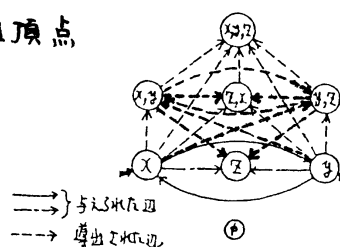
図6 自明な辺を明示しない閉包グラフ
