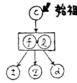
擬似推移的縮約図
