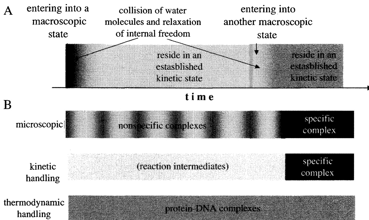
図1. 反応速度論の基盤 A: 分子が2つのkinetic stateを経験する例。グラデーションはShufflingをあらわし、hatchは転移過程そのものに要する時間。B: DNA結合タンパク質が、DNA上をnonspecific sites上を一次元的に拡散して、specific complexになる場合の物理的仮定（上）、反応速度論での表現（中）、熱力学での表現（下）。
