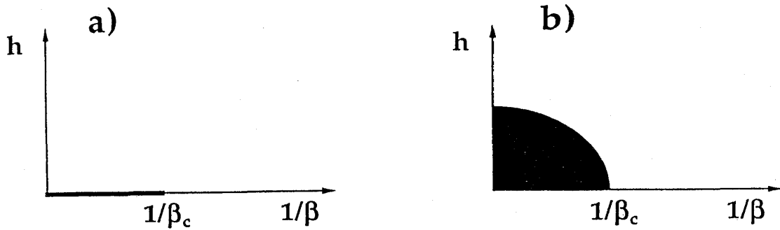
図4 ランダム磁場がかかったときに、長距離秩序が即座に破壊される場合(a)と、しばらくは残る場合(b)の相図。網をかけた部分が、長距離秩序のあるパラメータ領域を表す。Imry と Ma は、 1 < d \leq 2 で a) が、 d > 2 で b) が起こるとした。しかし Parisi と Sourlas によれば、 1 < d \leq 3 で a) が、 d > 3 で b) が起こるという。なお磁場が規則的に振動していて平均が0であれば、全ての d > 1 で b) が起こる事が知られている。
