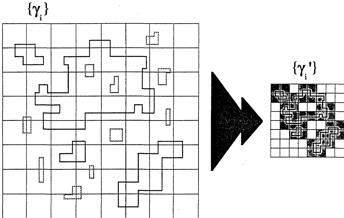
図 6 \{\gamma_i\} の l 以下のスケールのゆらぎをならして、くりこまれた contours の集まり \{\gamma'_i\} をつくる。先ず格子を一辺 l の正方形に分割する。広がりが l 以下の contours (図中点線で示した) を消し去った後、全体を 1/l に縮小する。最後に、右図で長さが 1 以下の構造を無視して、網かけで示したような新しい contour を得る。
