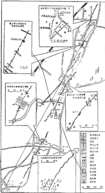
唐山地震震害区地震断層分布図
