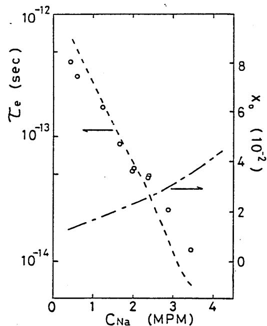
図 5 Na-NH 3 中の元/マー電子の \tau_c (o) と \tau_c (---)
