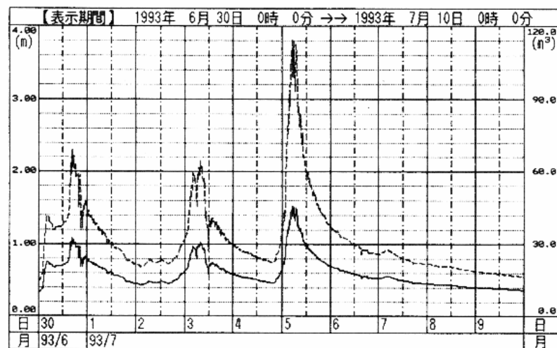
図—2 水位・流量記録をコンピューター表示した一例
