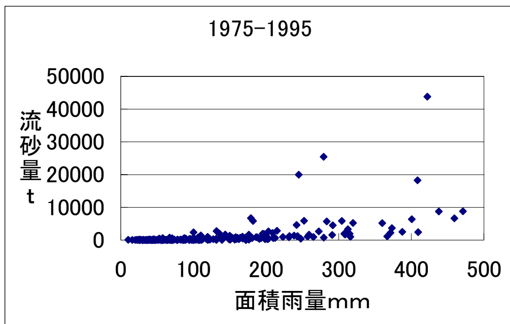
図—6 流砂量と降雨量の関係（1975.4～1995.12）
