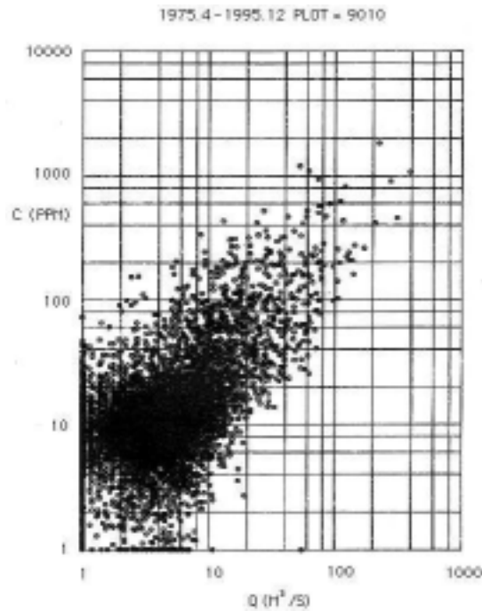
図—10 流量と濃度の関係
