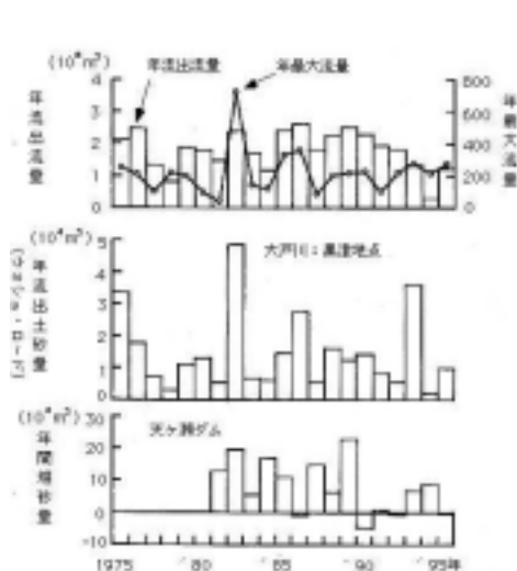
図—12 黒津地点の年流出流量・年最大流量 天ヶ瀬ダムの年間堆砂量（1995）
