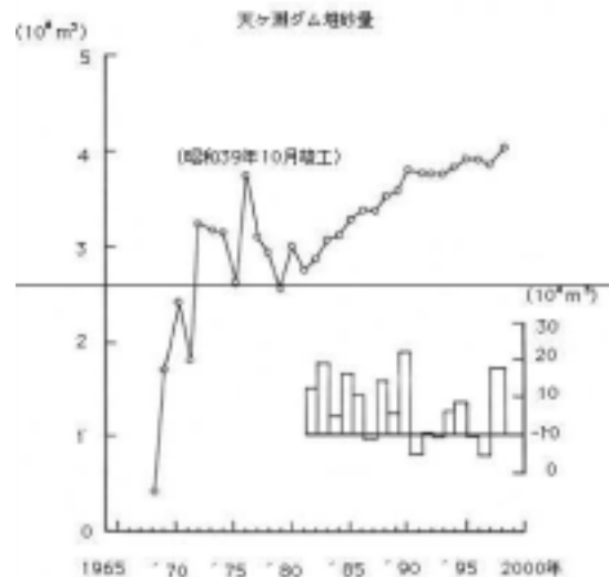
図—13 天ヶ瀬ダムの累積堆砂量と 年間堆砂量（1998）
