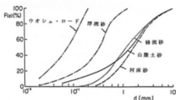
図—3 土砂の粒度分布（村本ら 1982）
