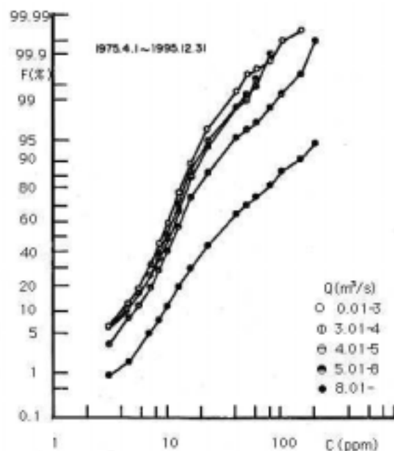
図—9 濃度の頻度分布図
