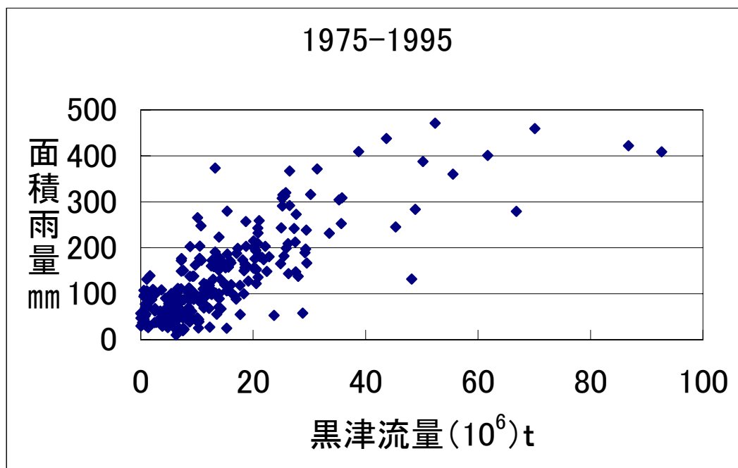
図—4 雨量と流量の関係（1975.4～1995.12）
