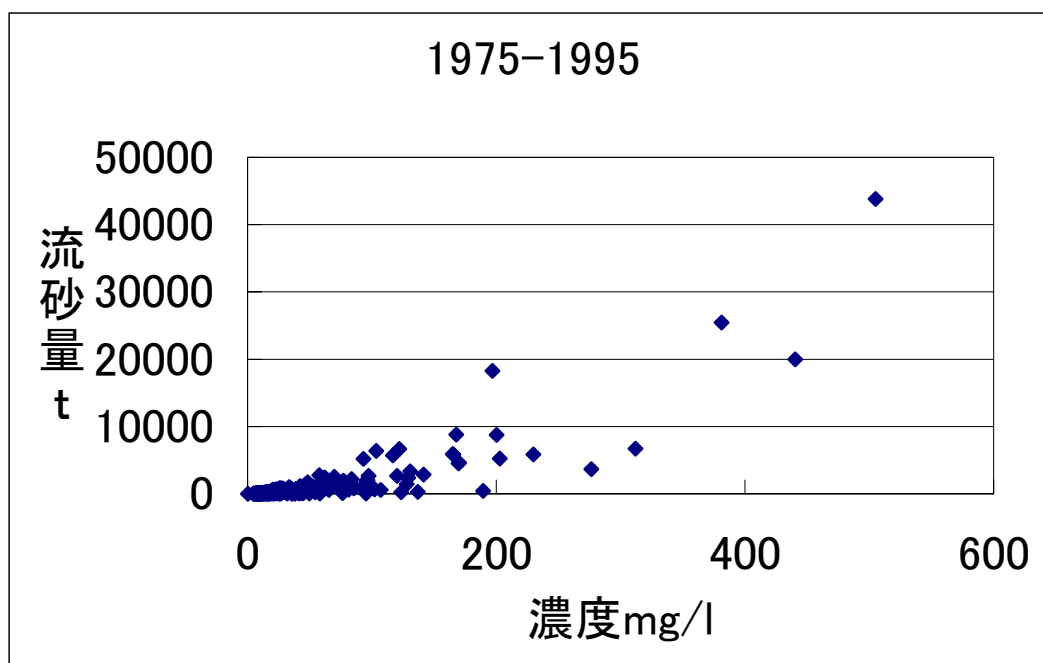
図—7 流砂量と濃度の関係（1975.4～1995.12）
