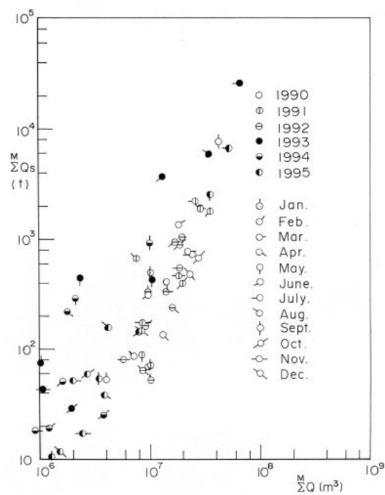
図—8 流量 Q と流砂量 (ウオシュ・ロード) Q_s の月別変化
