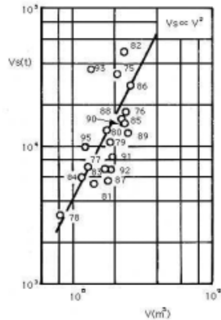
図—11 年流量とウオシュ・ロードの総量
