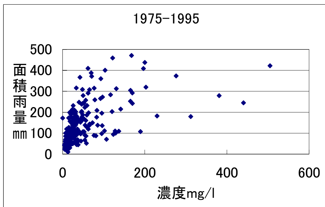
図—5 降雨量と濃度の関係（1975.4～1995.12）
