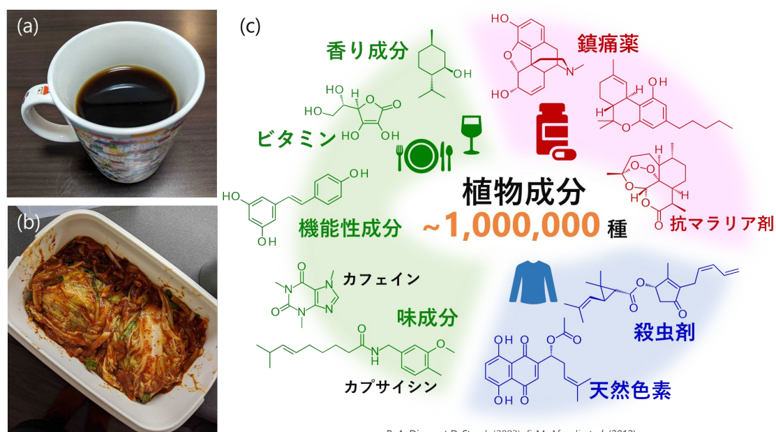
図 1：生活に身近な植物成分。(a) 覚醒成分カフェインが含まるコーヒー。(b) 辛み成分カプサイシンが含まれるキムチ。(c) 植物成分の化学構造と機能・用途の例
