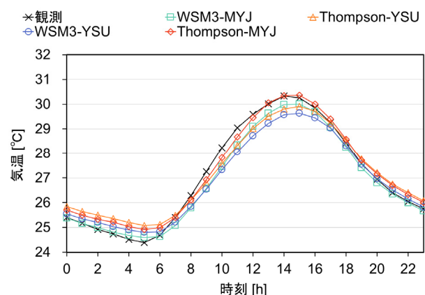
図 2：時刻別 1 ヶ月平均+10 年平均気温（7 月）
