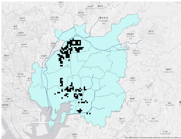
図7 1時間降雨量50mmの場合の浸水域の推定 (水色：名古屋市内、黒色：浸水域)
