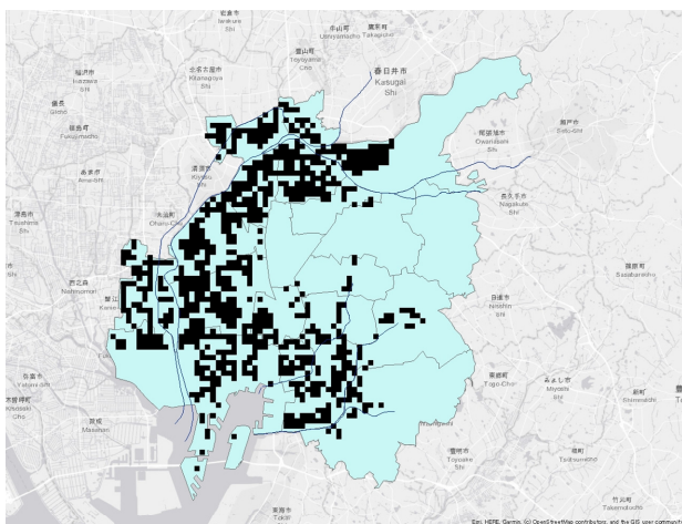
図8 1時間降雨量80mmの場合の浸水域の推定 (水色：名古屋市内、黒色：浸水域)
