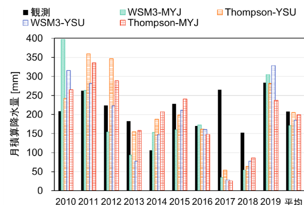
図 3：月積算降雨量（7 月）
