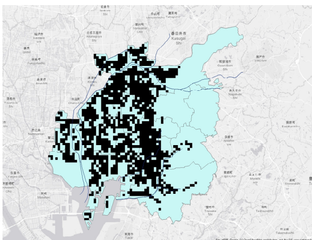
図9 1時間降雨量80mmの場合の浸水域の推定 (水色：名古屋市内、黒色：浸水域)
