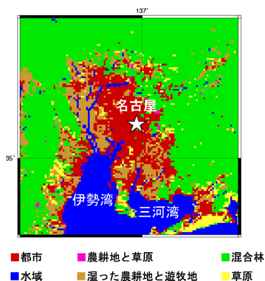
図 1：対象地域（名古屋都市圏）の土地利用分布
