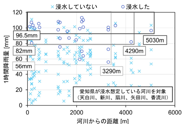
図 6 河川からの距離と降雨量の関係
