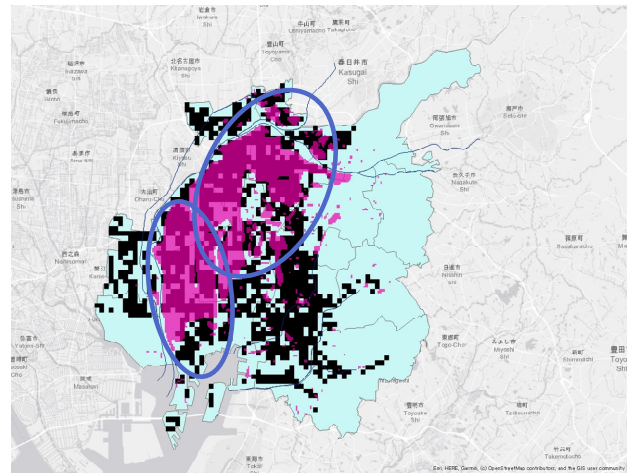
図10 過去の豪雨（平成20年8月末豪雨）時の 実際の浸水域と推定された浸水域（図9）の比較 （青枠：当該の過去の豪雨で90mm程度の降雨 が生じた範囲）
