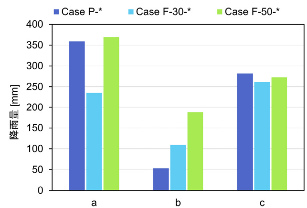
図5：月積算降雨量（7月）
