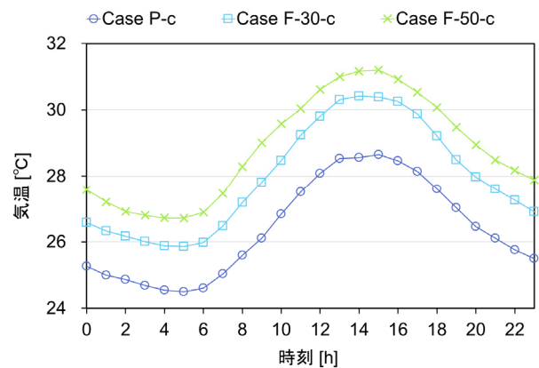
図4：時刻別1ヵ月平均気温（7月）
