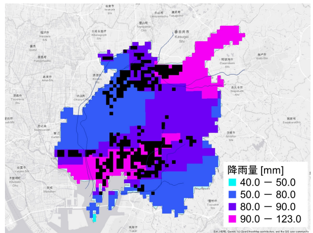
図11 将来気候下の浸水域の推定事例 (黒色：浸水域)
