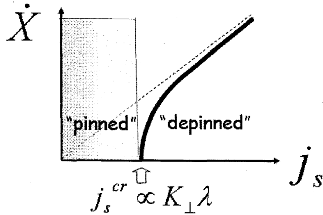
図 12: スピントルクによる磁壁の速さとスピンの関係。臨界電流値は困難軸異方性 K_{\perp}\lambda できる。
