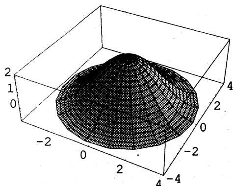
固有値 (\nu_1^{(0)})^2 の固有関数
