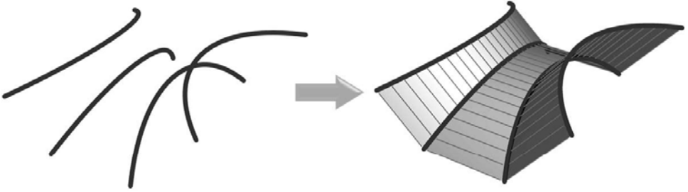
図 2: 半離散曲面の可視化．区分的な線織面 R_k(s, t) の貼り合わせにより，半離散曲面を可視化する．
