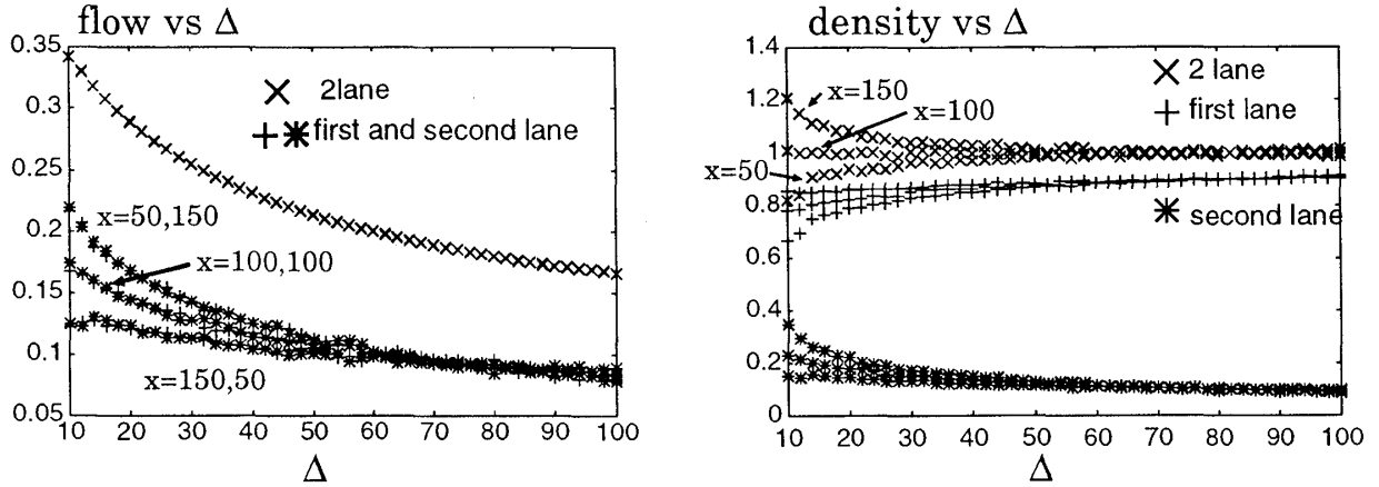
図8：レーンチェンジのバイアス \Delta に対する密度と流量。左が流量で右が密度。 \Delta の値が小さいところでは密度は両レーンとも位置に比例して大きくなるが、 流量の方は1レーン目が位置に反比例するのにに対し、2レーン目は比例する。
