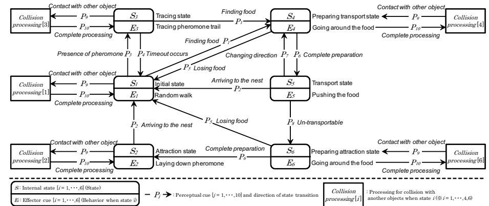
図1 フェロモン・コミュニケーションを用いて協調運搬をするための群行動アルゴリズム Fig.1 Algorithm for cooperative transportation using pheromone communication
