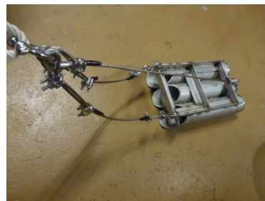
写真 5: ステンレス製採砂器
