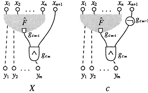
図 1: F(x_1, \dots, x_n) に対して構成される BCI のインスタンス X と c .
