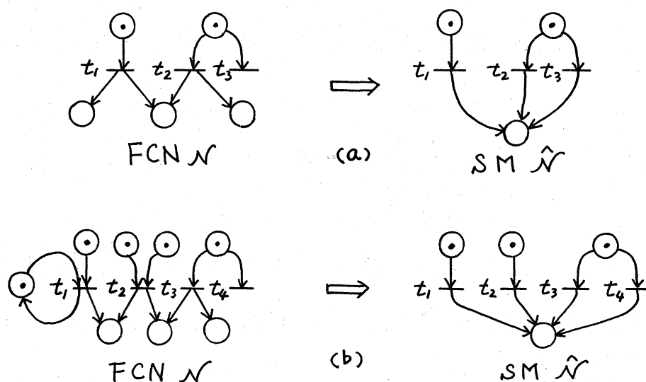
図1 FCN \mathcal{N} から SM \hat{\mathcal{N}} への変換
