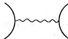
第1図 粒子交換による重力相互作用。
