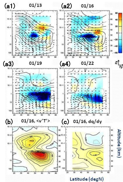
図 4: (a)2009 年 1 月 13, 16, 19, 22 日の帯状平均東西風(コンター), E-P flux(ベクトル), DF(カラー)の緯度高度断面図. コンター間隔は 10 m/s, ユニットベクトルは 10^{-1} \cdot 10^2 hPa の領域で F_y: 2 \times 10^6 , F_z: 2 \times 10^8 (kg/s 2 ), これ以上の 10^1 \cdot n \cdot 10^2 \cdot n hPa ( n=1-3 )の領域ではスケールを 5n 倍, 10^{-3} \cdot 10^{-2} hPa の領域では 25 倍している. DF の単位は m/s/day. (b)東西風と気温の波の積を帯状平均したもの \overline{v'T'} で, コンター間隔は 50 m 2 /s 2 . (c)準地衡風渦位の南北勾配 \partial \bar{q} / \partial \phi で, \Omega で割った値を示している. E-P flux, DF, \overline{v'T'} は東西波数 1-3 の成分のみで描いている.
