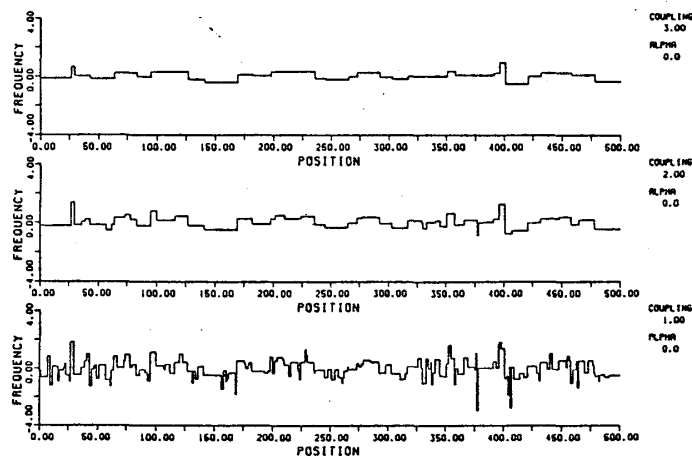
図4. \alpha=0, d=2 の同一振動数フラスター (隣りあう格子点間の振動数の差異がないとみなされる場合に格子点間にボンドを描いた)
