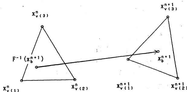
図3 重心に移動してくる粒子
