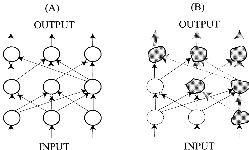
図 1: (A) Boolean Circuit の例。それぞれの素子では \wedge (and) や \vee (or) などの基本 Bool 演算やその組み合わせ演算を行う。出力が複数ある場合には同一の出力結果が次の全ての素子へとつながる。(B) 右下の素子で発生したエラーが時間とともに伝搬してしまう。
