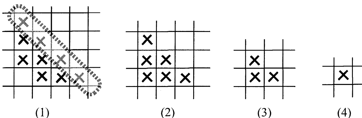
図 3: Toom のセルオートマトンがエラー修正を行う様子。×印がエラーの起こったセル。(1)では点線で囲まれたセルが次のステップでエラー修正される。以下 (2)~(4) まで左下方向に向かって順次エラーが修正され、最後のステップでは完全にエラーが消滅する。
