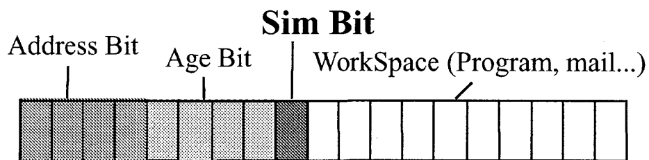
図 7: セルの状態の 2 進数表記。セルの状態数を 2^k とすると、 k bit で表現する。
