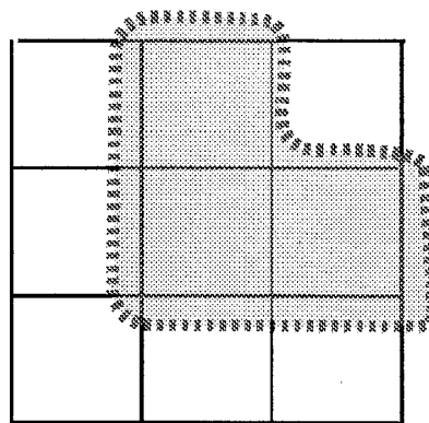
図 2: Toom の 2 次元セルオートマトン。中央が自分のセル。点線で囲った部分のセルの状態を見て多数決を取って次の状態を決める。
