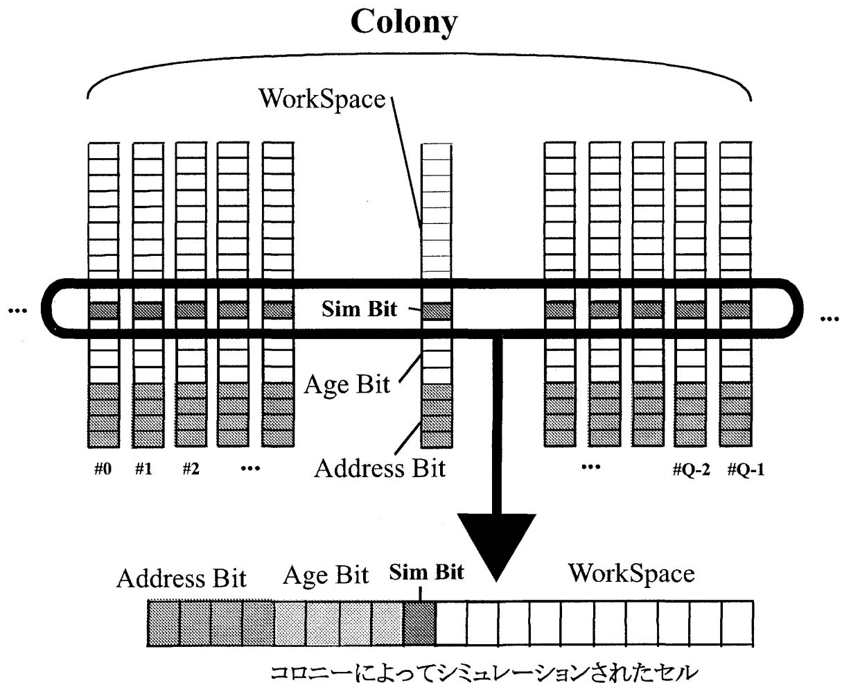
図 8: コロニーによる自己シミュレーション。各セルの状態 bit 列を縦に表記してある。#記号はセルのコロニー内でのアドレス。Sim Bit を繋ぎ合わせて眺めると、あたかもひとつのセルであるかのように振舞う。このシミュレーションされたセルの Sim Bit を再び繋ぎ合わせると、今度はコロニーのコロニーによる自己シミュレーションが実行されている。
