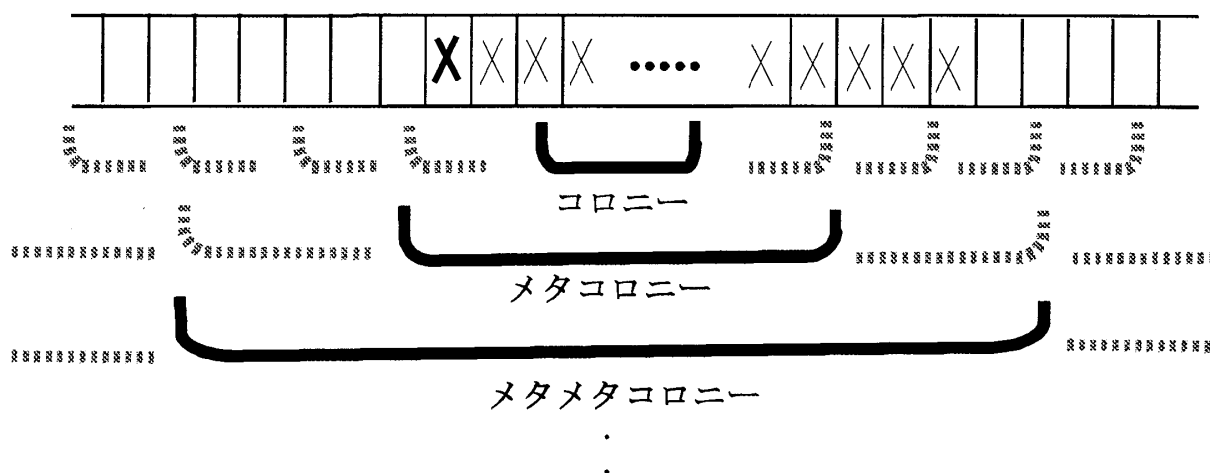
図 6: コロニーはセルの集合体であり、エラー処理はコロニー単位で行われる。しかし、ひとつのコロニー内で処理できないような広範囲にわたるエラーにはコロニーのコロニー (メタコロニー) 単位で処理が行われる。さらにメタコロニーでも処理できなければメタメタコロニーが... 無限に再帰的な連鎖は続く。
