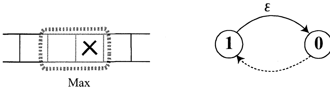
図 5: 1次元方接触モデル。自分と左隣のセルで大きい方の値を採用する。右図の状態遷移図に示したように、状態 1 は確率 \epsilon で遷移する可能性があるが、状態 0 は普通の状態遷移規則にしたがって遷移するときだけ状態 1 になる。
