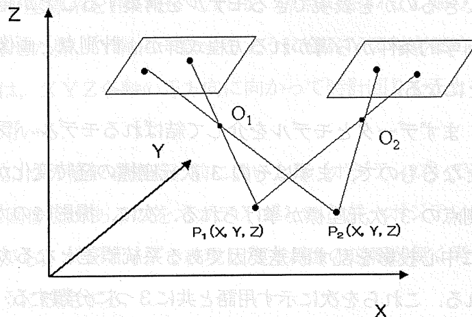
図 2.1.1 立体画像構築の原理
