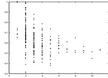
図 6 所属アカウント数とアクセス権限適合率の相関 (100 ユーザ)
