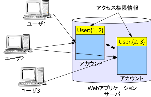
図 3 複数のアカウントを利用する手法
