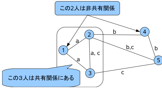
図 5 データ共有関係グラフ
