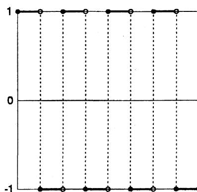
w_4(x)
