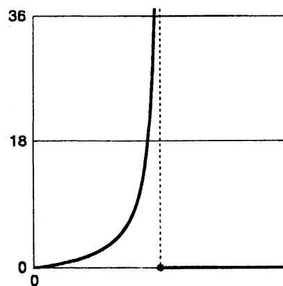
w_4(x)
