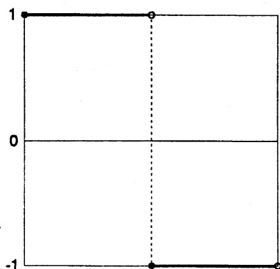
w_1(x)
