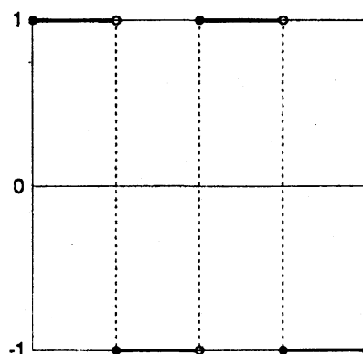
w_2(x)
