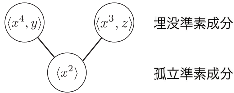
図 2: $\langle x^4, x^3y, x^2yz \rangle$ の準素成分のグラフ
