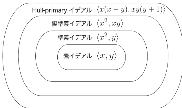
図 5: イdealの概念の関係
