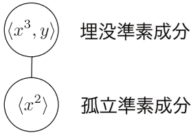
図 1: $\langle x^3, x^2y \rangle$ の準素成分のグラフ
