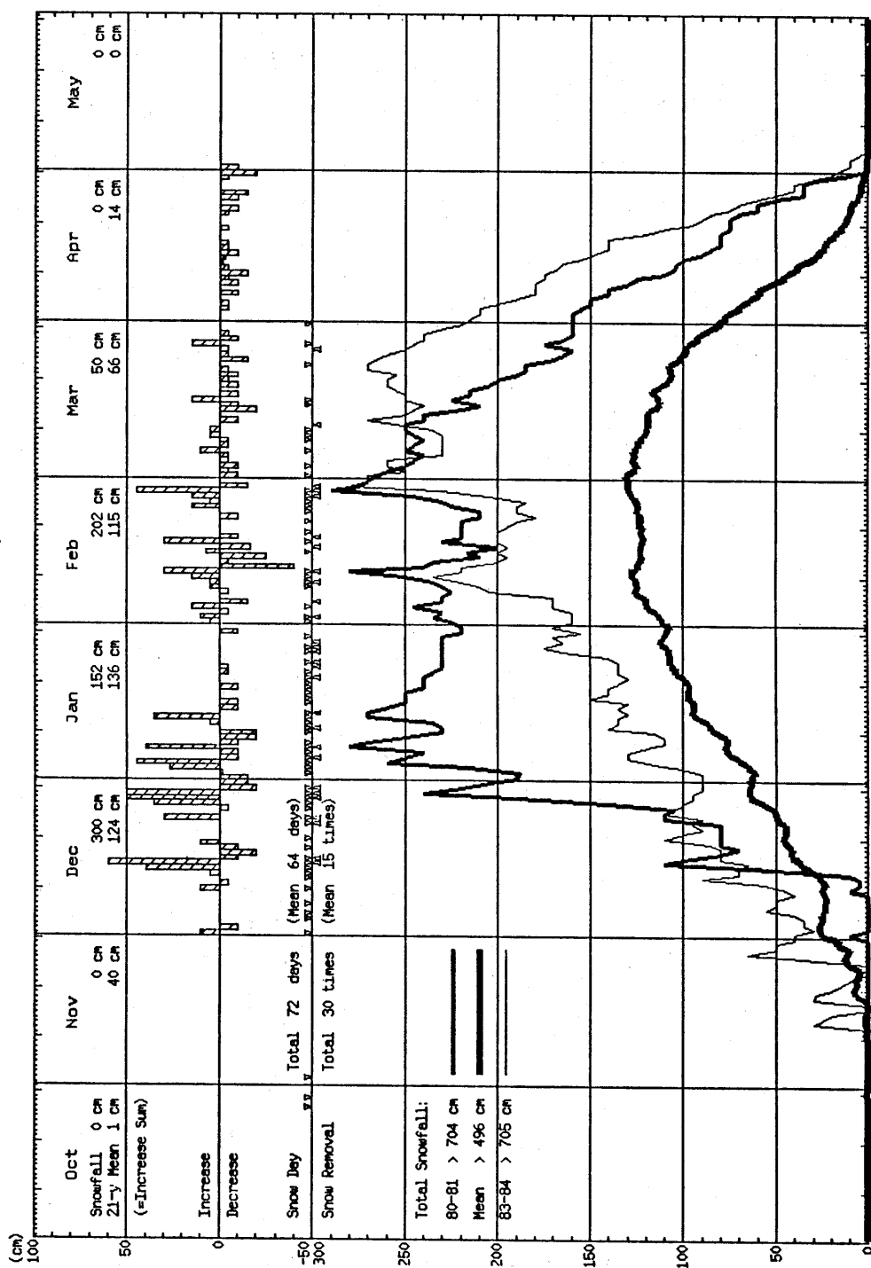
図4. 豪雪時の積雪パターン。「56豪雪」と「59豪雪」及び平年.
