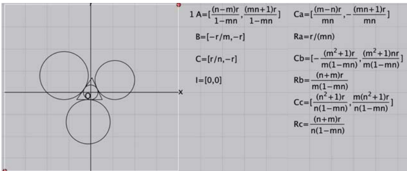
図 9: 亨円と3傍接円
