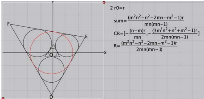
図 11: 4 円径の和 sum と内接円の半径 R
