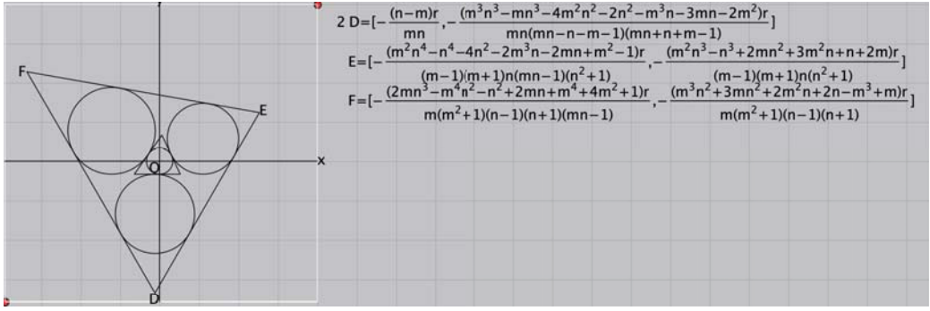
図 10: 共通外接線と三角形 DEF
