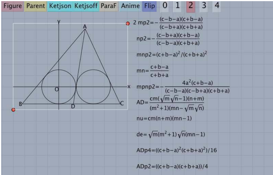
図 8: AD^2 を a, b, c で表す
