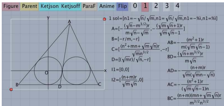
図 7: m, n, r による結果
