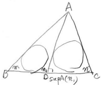
図 6: ラフスケッチ
