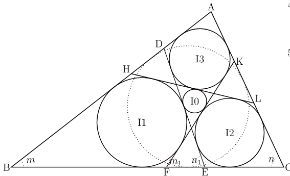
図 14: HL, DE, KF に接する円 I0
