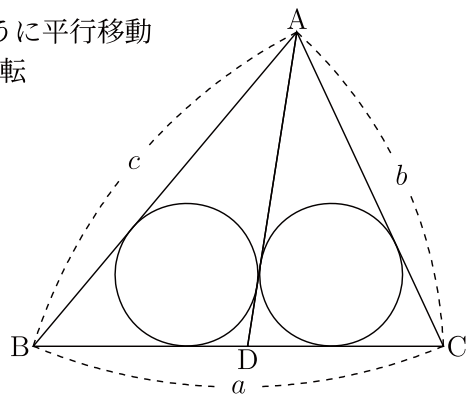
図 3: AD を a, b, c で表す (問 2.2.5)
