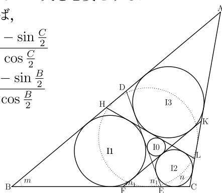
図 15: 鈍角三角形の場合
