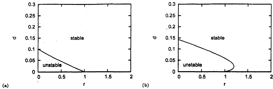
図 1: Prey-Preator 系における内部固定点の安定性解析の結果. (a) k = 2 の場合, (b) k = 3 の場合.
