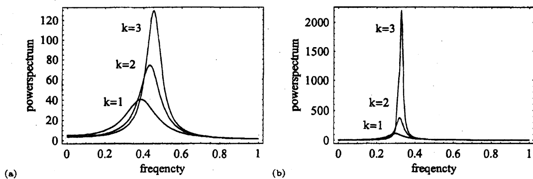
図 2: Prey-Preator 系におけるパワースペクトルを線形近似で計算したもの. パラメータは (a) r = 1, d = 0.2 , (b) r = 1, d = 0.1 . \sqrt{N} 倍してスケールしていることに注意.
