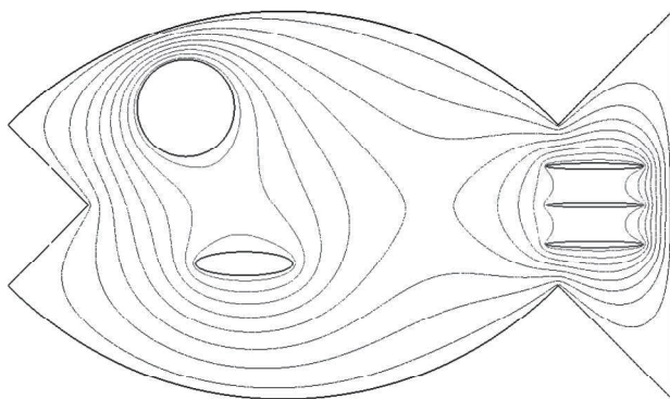
Figure 1: 平面領域上の調和関数の等高線図 (FreeFEM++で作成). 境界の凹んだ角 (たとえば魚の口) のまわりでは減衰が急になり, 領域内部のことばで言えば“たるみ”が生じている.
