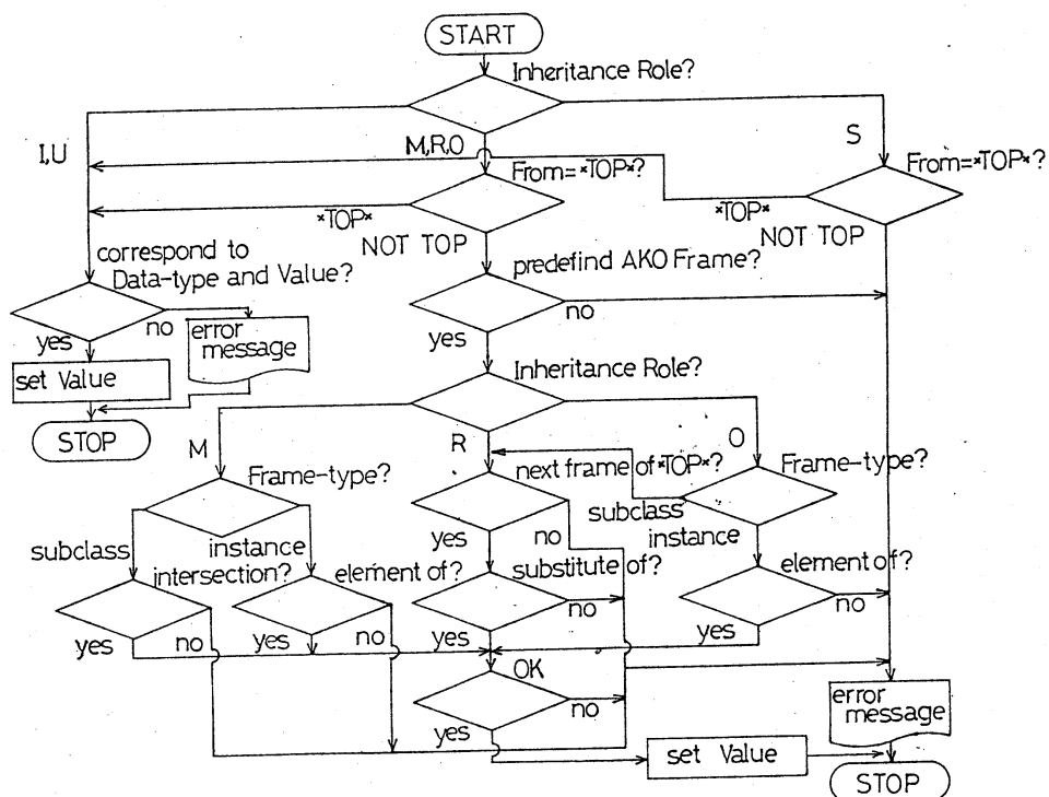
図7 スロットの値を設定する操作に関するチェックの流れ
