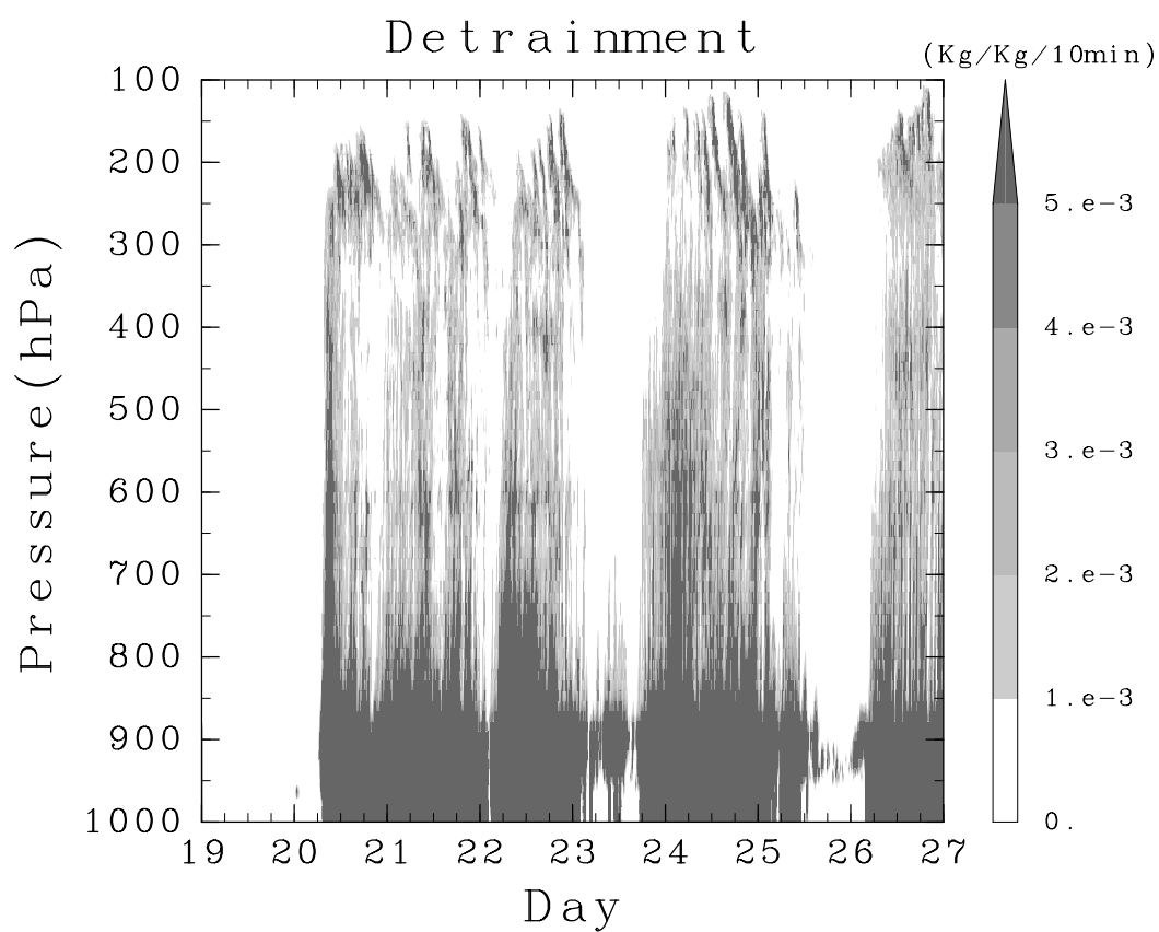
Figure 4 領域平均したトレーサ T_2 のデトレイメント量の鉛直分布の時間変化. 期間は, 12 月 19 日~27 日. デトレイメント量は, 10 分間のトータル量. 1.0 \times 10^{-3} \text{ kg} \cdot \text{kg}^{-1} \cdot 10 \text{ min}^{-1} 毎に色を塗り分けている.
