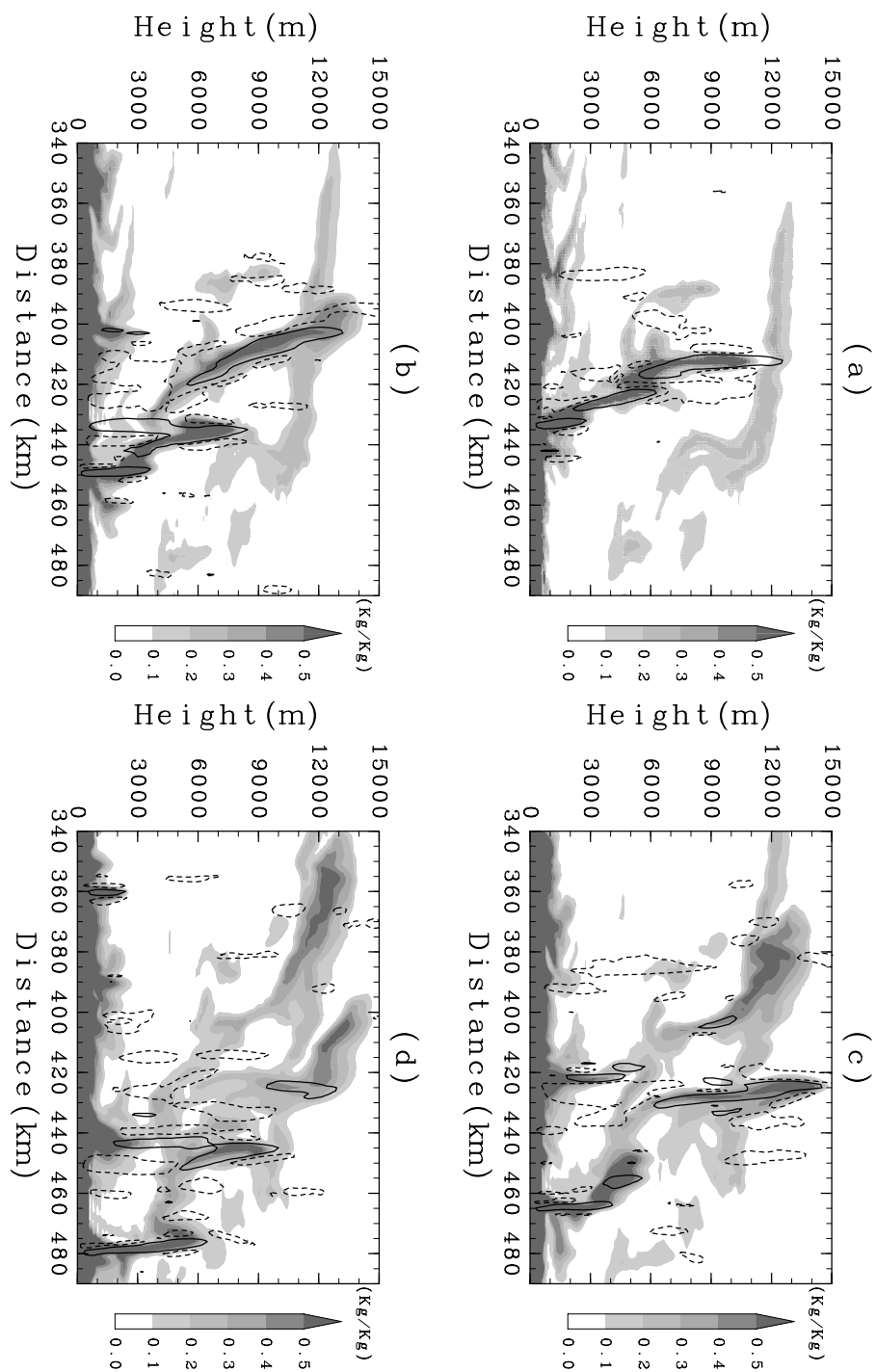
Figure 5 モデル内で計算されたトレーサ T_3 の積雲対流による上方輸送の様子。それぞれの図の時間間隔は 30 分である。色の塗りわけは、トレーサ混合比 0.1 \text{ kg}\cdot\text{kg}^{-1} 毎に行っている。実線のコンターは、 1.5 \text{ m}\cdot\text{s}^{-1} の上昇流を示す。破線のコンターは、 0.5 \text{ m}\cdot\text{s}^{-1} の下降流を示す。
