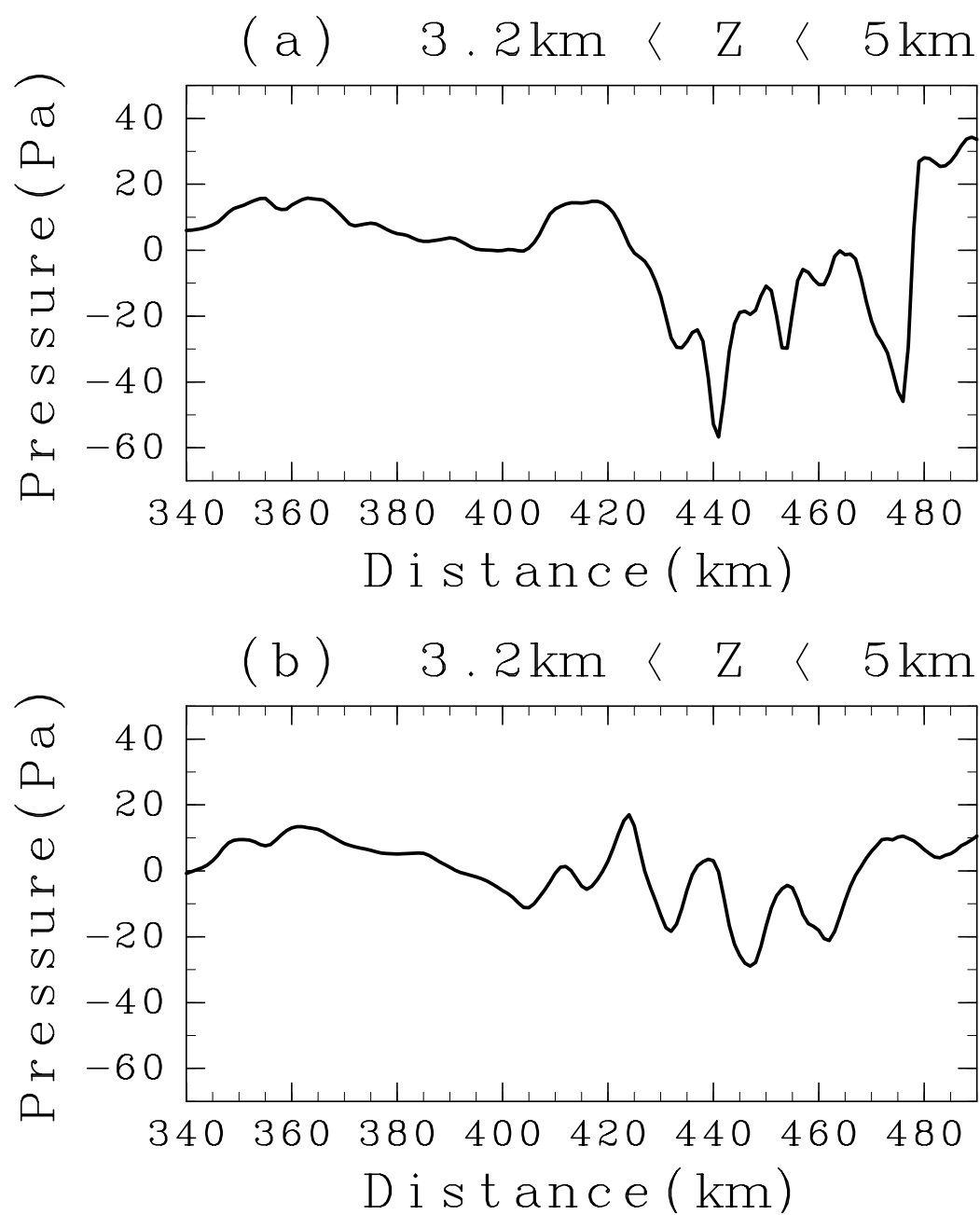
Figure 12 圧力の水平平均からのずれを高度 3.2 km と 5.0 km で平均した水平分布図. (a) と (b) はそれぞれ, 図 5(d) と 図 10(d) に の対流システムに対応している.
