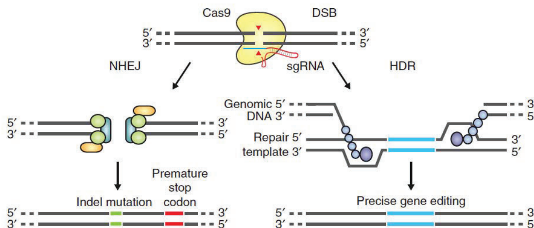
図5 CRISPR/Cas9 システム 6)
