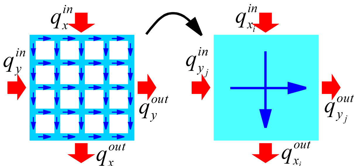
Fig.4 要素集約型氾濫水伝播モデルの概要
