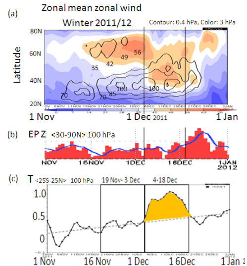
図 1. (a) 0.4hPa(等値線)と 3hPa(彩色)の帯状平均東西風の緯度－時間断面。(b) JMA による 100hPa 北半球（30-90 度）平均 E-P フラックスの鉛直成分。(c) 熱帯域（25S-25N）で平均した 100hPa の気温偏差。
