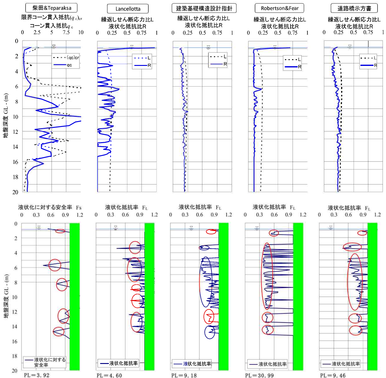
図-6 RI コーン貫入試験結果に基づいて算定した、5 種類の手法による液状化抵抗値 R と地震によって動員される繰返しせん断応力比 L の深度方向分布と液状化危険度評価結果
