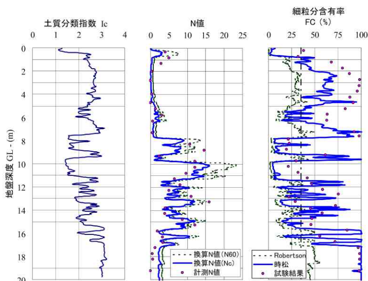
図-4(a) RI コーンによる土質分類指数，換算 N 値，粒分含有率 (調査地点 No.1)
