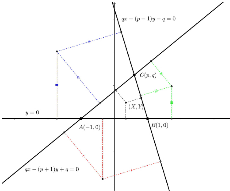
図 3: 3つの頂点を通る直線から等距離にある点
