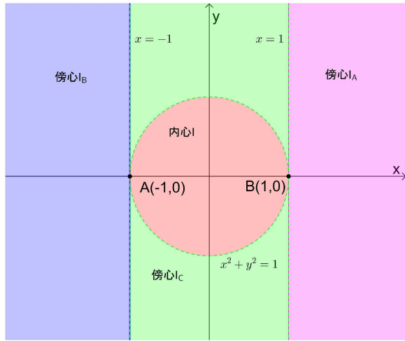
図 6: 内心 I と 3 つの傍心 I_A , I_B , I_C が存在する領域
