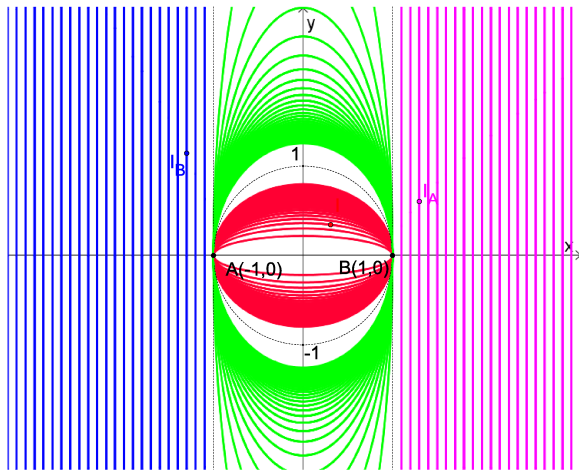
図 5: 内心 I と 3 つの傍心 I_A , I_B , I_C の軌跡の変化の様子
