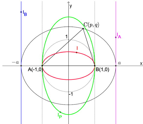
図 2: 内心 I と 3 つの傍心 I_A , I_B , I_C の軌跡
