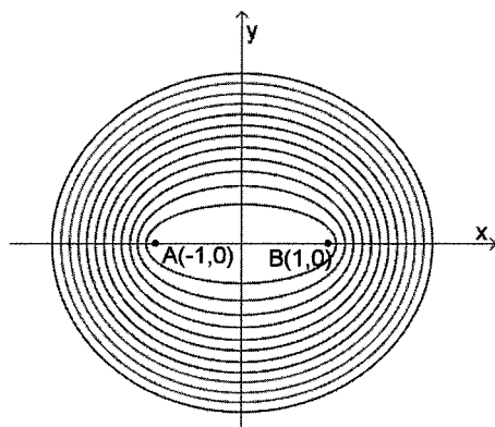
図 4: 楕円の変化の様子
