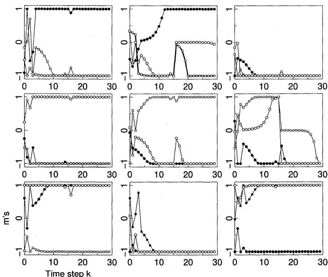
図 3: ランダムな初期状態から出発して正解に達した例。各ステップで強制的に二値化 (急冷) して「答え合わせ」をしてみると、20 ステップ目で正解のベージンに入ったことがわかる。
