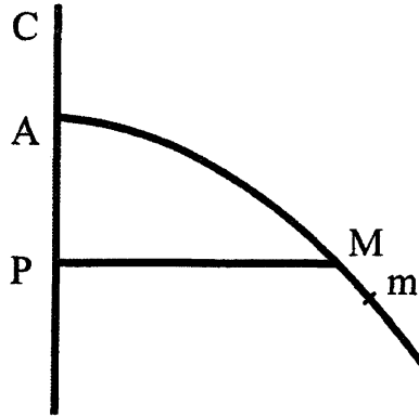
図1 一定の重力による運動
