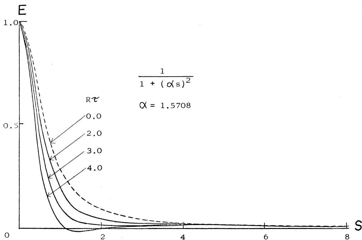
図 6: エネルギー・スペクトルの時間的変化の比較。 R = 100 .
