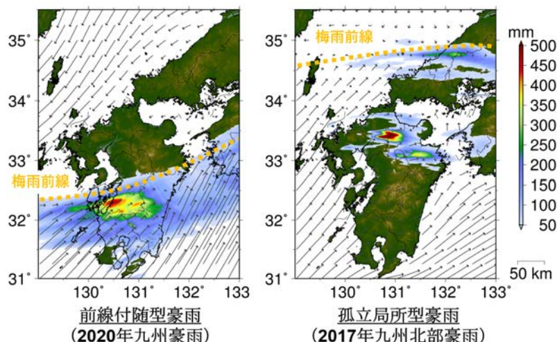
図2 梅雨前線に伴う線状対流系豪雨の2つのタイプ
