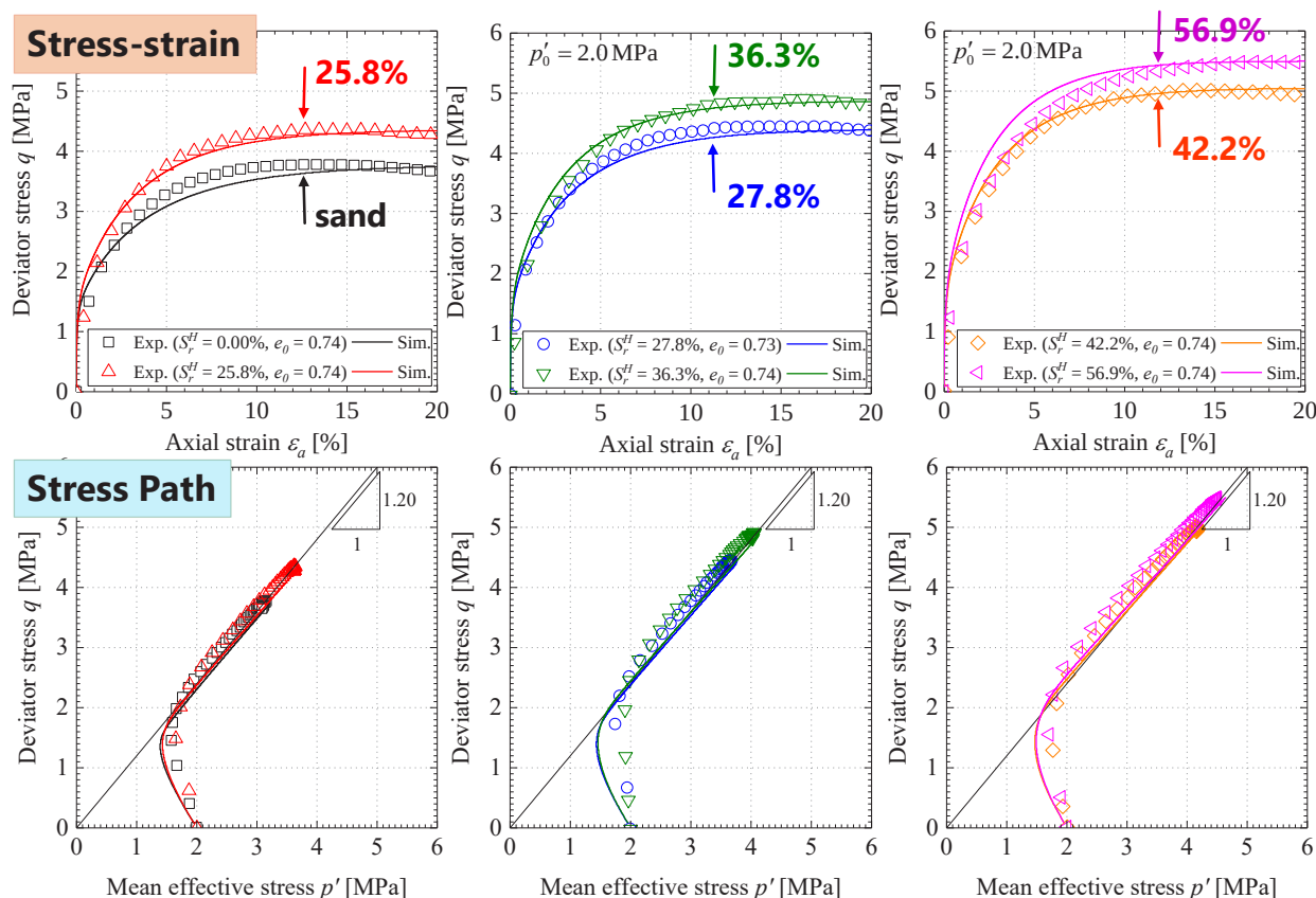
図4 \text{CO}_2 ハイドレート含有地盤の非排水三軸圧縮試験結果（シンボル）と構成式による計算結果（実線）の比較
