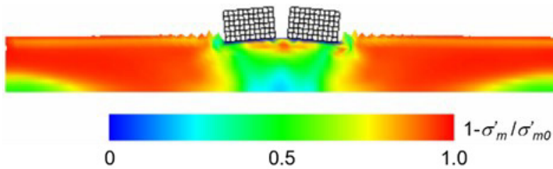
図7 二次元弾塑性有限要素法による液状化地盤上におけるボックスカルバートの動的解析
