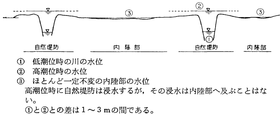
図5 海岸平野の水文環境
