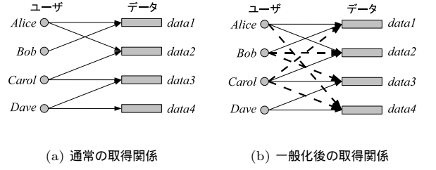
図 4 データ取得情報からの権限情報推定
