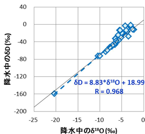
図2. 瀬戸臨海実験所における降水の \delta -ダイアグラム。黒線はグローバルな天水線 ( \delta D = 8 \times \delta^{18}\text{O} + 10 )、青の点線は瀬戸臨海実験所におけるローカルな天水線を示す。
