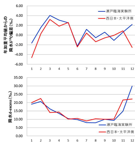
図3. 瀬戸臨海実験所と IMWG によって得られた西日本・太平洋側 (全 20 地点) における降水中の \delta^{18}\text{O} (上段) と d-excess (下段) の季節変化。
