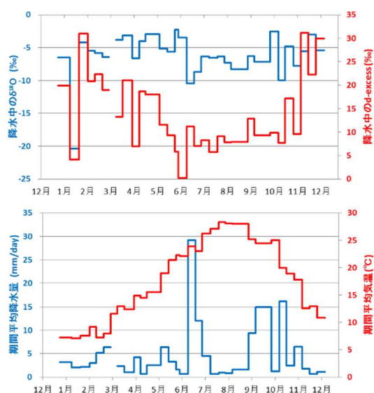
図1. (上段) 瀬戸臨海実験所における降水中の \delta^{18}\text{O} (青線) と d-excess (赤線) の季節変化。(下段) 同実験所における採水期間中の日降水量 (青線) と日平均気温 (赤線)。
