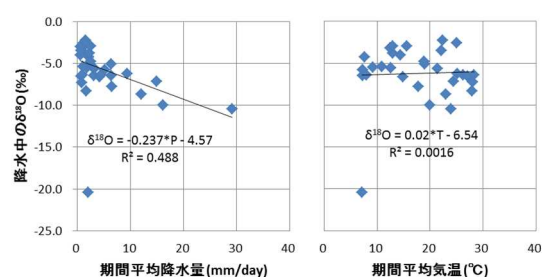
図4. 瀬戸臨海実験所における降水中の \delta^{18}\text{O} と期間平均した日降水量、または日平均気温との関係。回帰直線とその式、決定係数を示す。回帰直線の計算には、N-02 のサンプルは除外した。
