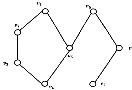
Fig. 2. Poset P
