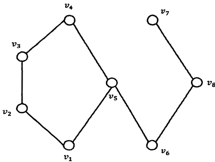
Fig. 10. Poset P_d
