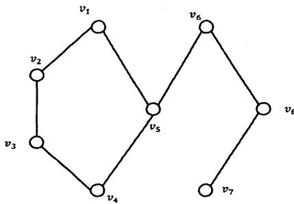
Fig. 8. Poset P
