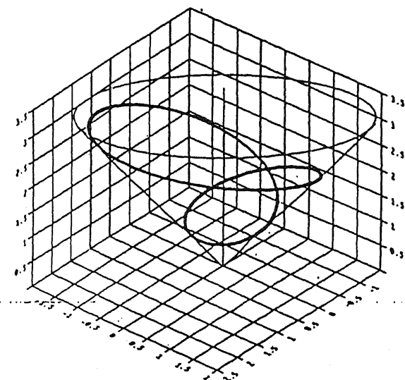
図3 2-fold Kepler型の軌道
