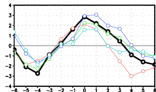
図5 年平均 F10.7 で回帰した各種諸量のラグ年に対する変化。横軸はラグ年。以下、赤線は DJF 平均した 1hPa 赤道の気温(2 倍: 単位 K)、黄緑線は 2hPa 面上 30-40 度平均した -dT/dy ( 5 \times 10^6 倍: 単位 K/m)、水色線は DJ 平均した PJO 指数の -PC2 (20 倍: 単位なし)、青線は JF 平均した PJO 指数の PC1(10 倍: 単位なし)、黒線は DJF 平均し
