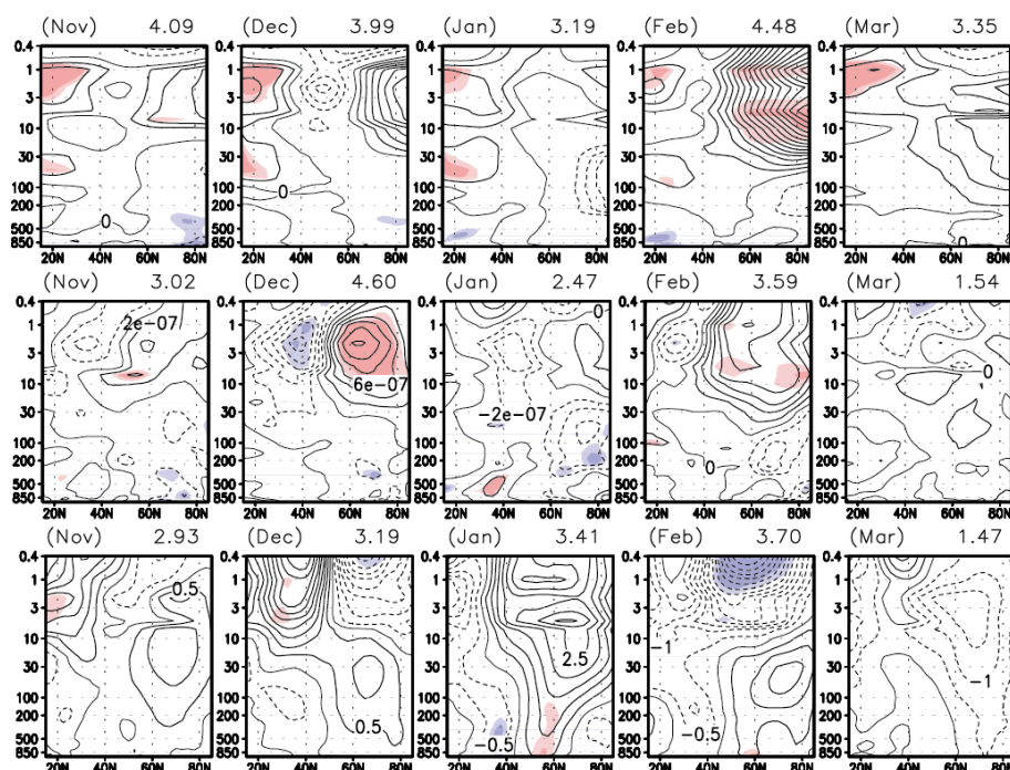
図2 年平均 F10.7 で回帰した 11 月から 3 月までの(上段)温度偏差場、(中段)温度場の南北勾配、(下段)平均東西風。横軸は緯度で 15N から 85N を、縦軸は気圧で表した高度であり、1000hPa から 0.4hPa を表す。コンター間隔は、温度場は 0.3K、温度の南北勾配は 2 \times 10^{-7} \text{K/m} 、東西風は 0.5m/s であり、濃い(薄い)ハッチは統計的に 98(95)% で有意である領域を表す。
