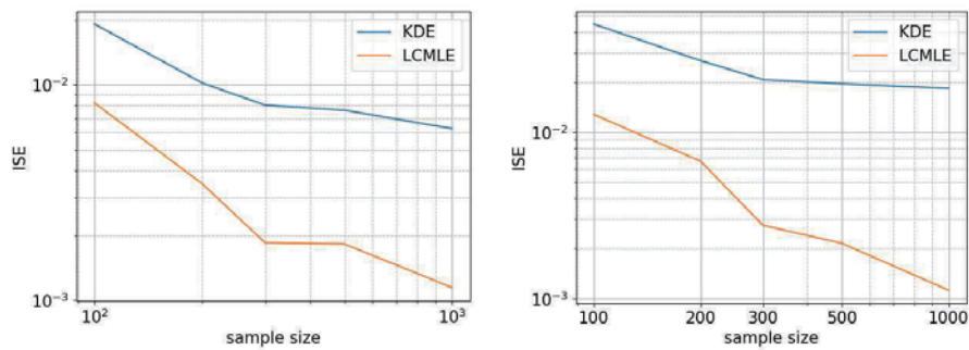
図 5 サンプルサイズ 100, 200, 300, 500, 1000 における平均積分二乗誤差. (左): ケース 1, (右): ケース 2. LCMLE は対数凹最尤推定量, KDE はカーネル密度推定量を表す.
