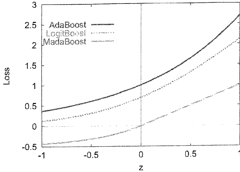
図 4: ロジスティックモデルに関連したロスのグラフ.
