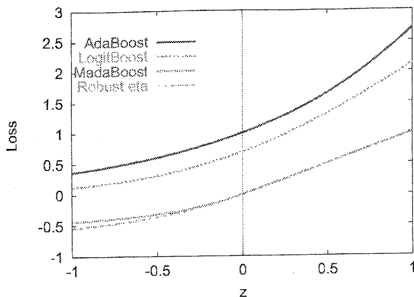
図 6: モスト B-ロバストな \eta -ブーストのロスのグラフ.
