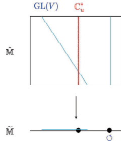
図 1 \mathbb{C}_u^* -作用
